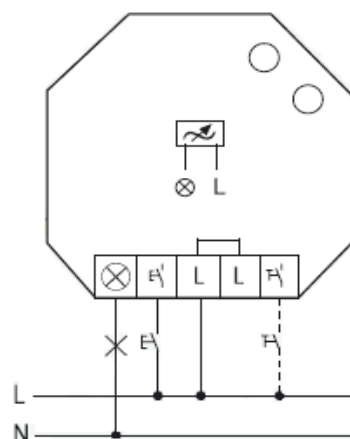
Koblingskjema
